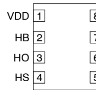
SOIC/DFN8
